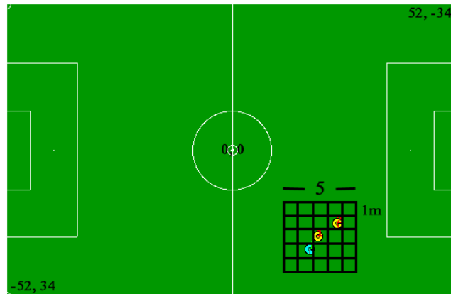
Abbildung 14: Eine „Situation“: Der RL-Spieler mit der Nummer 1 befindet sich an x=20 y=20 , der nächste Mitspieler an Stelle x=24 y=17 und der nächste Gegner an x=18 y=23 .
